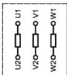
Рисунок 3 - Трехфазное электрооборудование с шестью выводами
